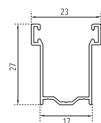
Guida in alluminio A28 17X27 mm
