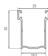
Guida in alluminio A30 19,5X30 mm
