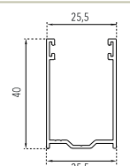
Guida in alluminio A40 25,5X40 mm
