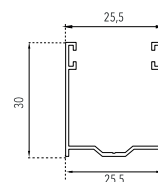
Guida in alluminio A27 25,5X30 mm
