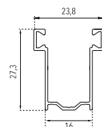
Guida in alluminio A16 16X27,3 mm
